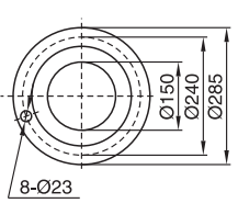
( Discharge Flange ) DN2
