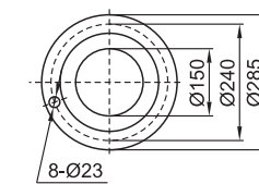
( Discharge Flange ) DN2
