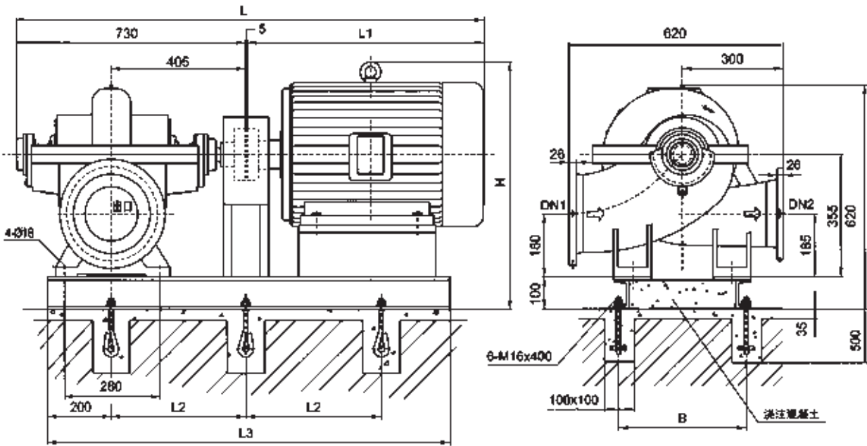
吸入法兰(Suction Flange)DN1及吐出锥管出口法兰 吐出法兰 ( Discharge Flange ) DN2
