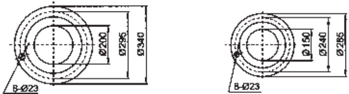
吸入法兰(Suction Flange)DN1及吐出锥管出口法兰 吐出法兰 ( Discharge Flange ) DN2
